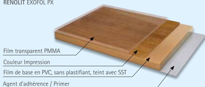
Structure schématique du film extérieur RENOLIT EXOFOL PX
